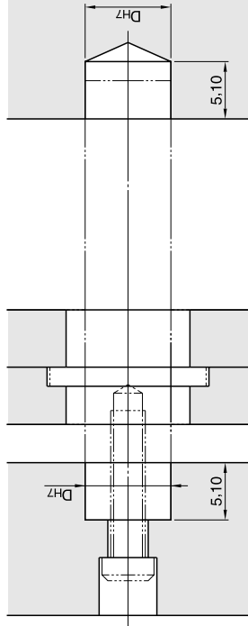
精密级推板导柱(EGH)适用
