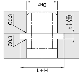
铜合金自润滑型推板导套(EGBZ)适用
