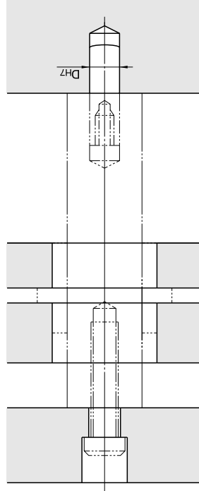
销定位精密级推板导柱(EGHC)适用
