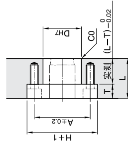
浇口套导向套适用
