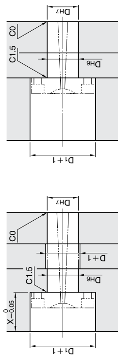
JIS A型浇口套适用
