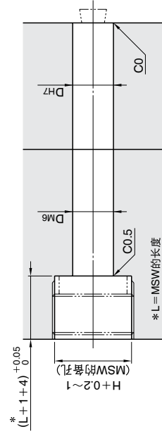
直杆型拉料销适用
