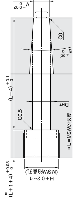
锥型拉料销适用
