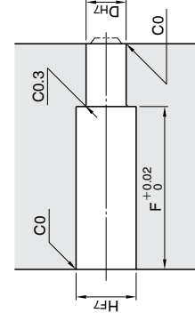
点式浇口套适用
