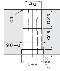
浇口锁料套(SLBH)适用
